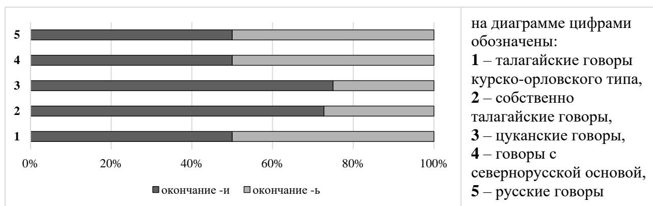
Диаграмма 20. Соотношение вариантов безударного окончания дат.п. ед. ч. 1 скл. существительных в говорах Воронежской области
