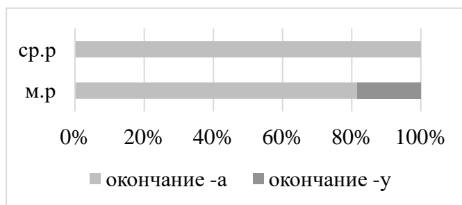
Диаграмма 26. Соотношение вариантных окончаний род. п. сущ. 2 склонения в цуканских говорах
