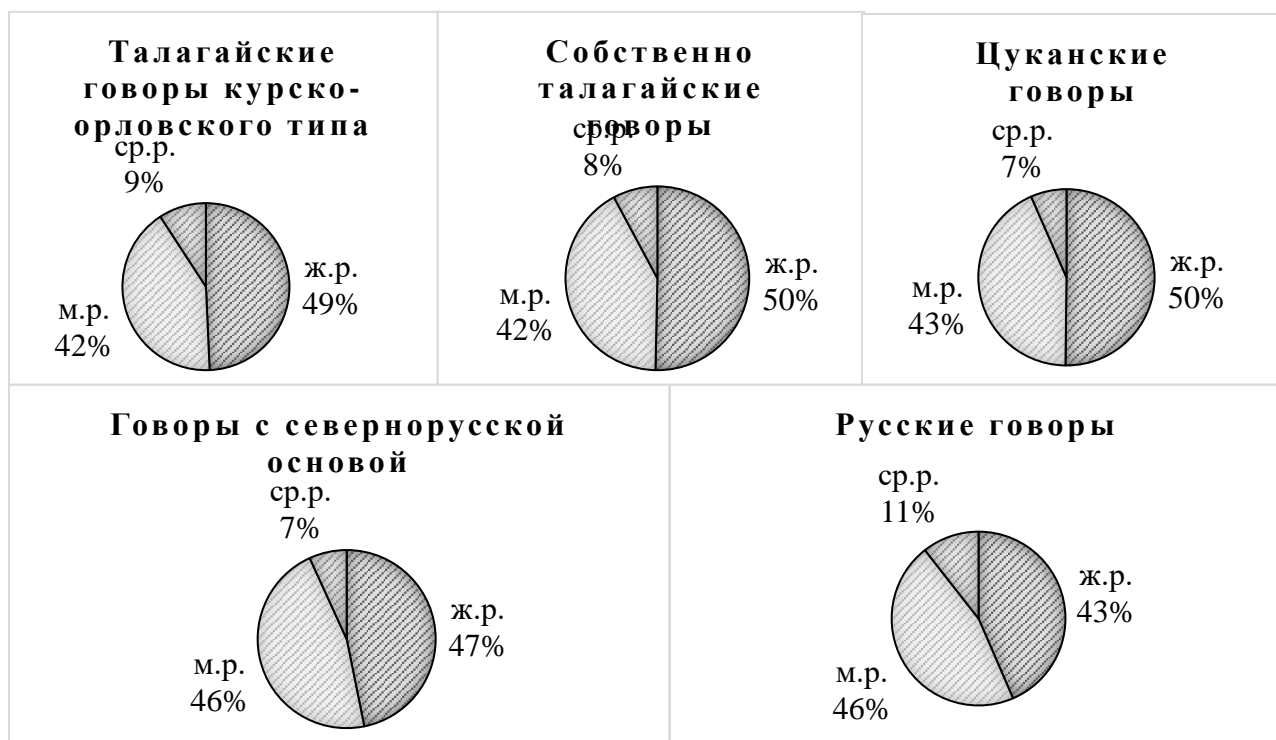
Диаграмма 9. Распределение существительных по родам в воронежских диалектах
