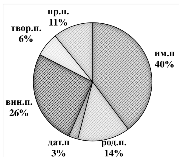
Диаграмма 11. Распределение существительных в ед.ч. по падежам в говорах Воронежской области
