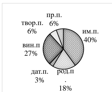
Диаграмма 35. Распределение существительных по падежам во мн.ч. в говорах Воронежской области
