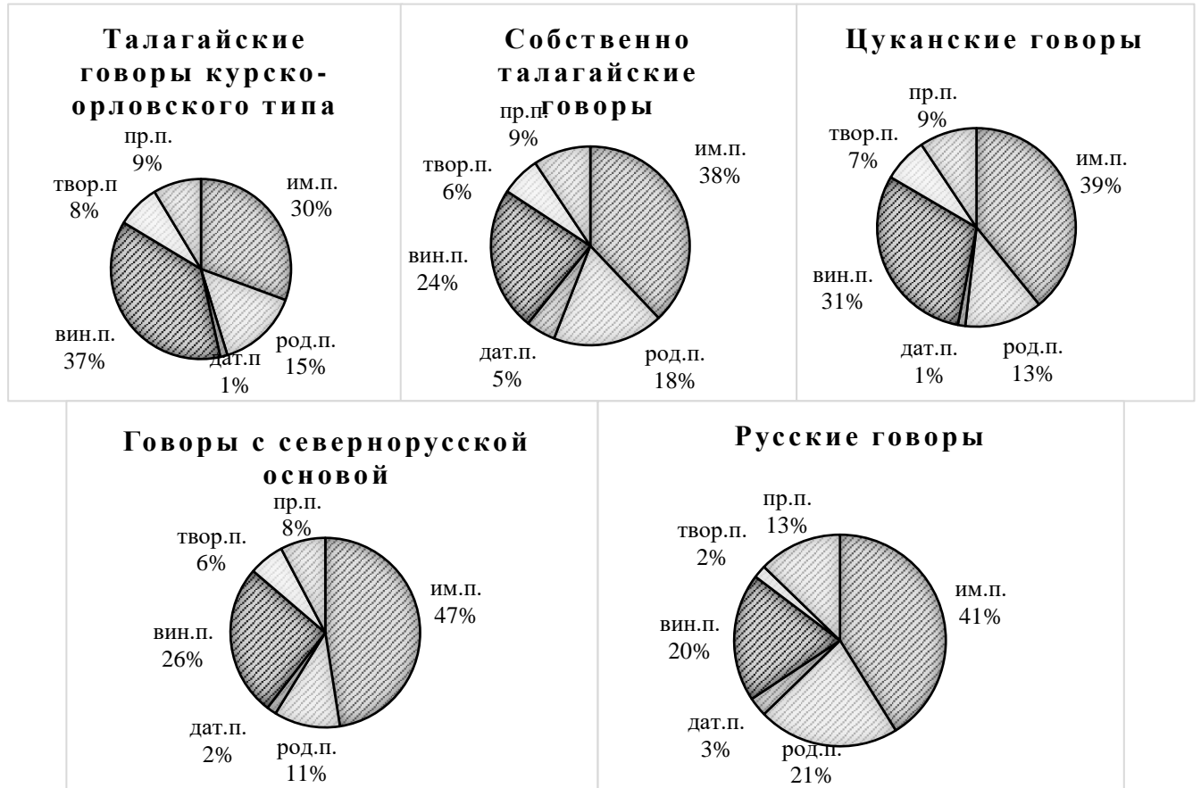
Диаграмма 14. Распределение существительных 1 склонения ед.ч. по падежам в говорах Воронежской области
