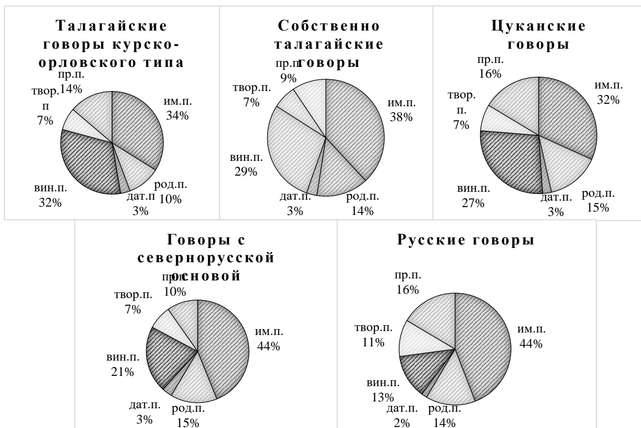
Диаграмма 22. Распределение существительных 2 скл. ед.ч. по падежам в говорах Воронежской области
