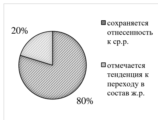
Диаграмма 5. Существительные ср.р. в собственно талагайских говорах
