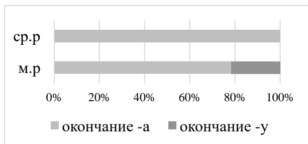
Диаграмма 25. Соотношение вариантных окончаний род. п. сущ. 2 склонения в собственно талгайских говорах
