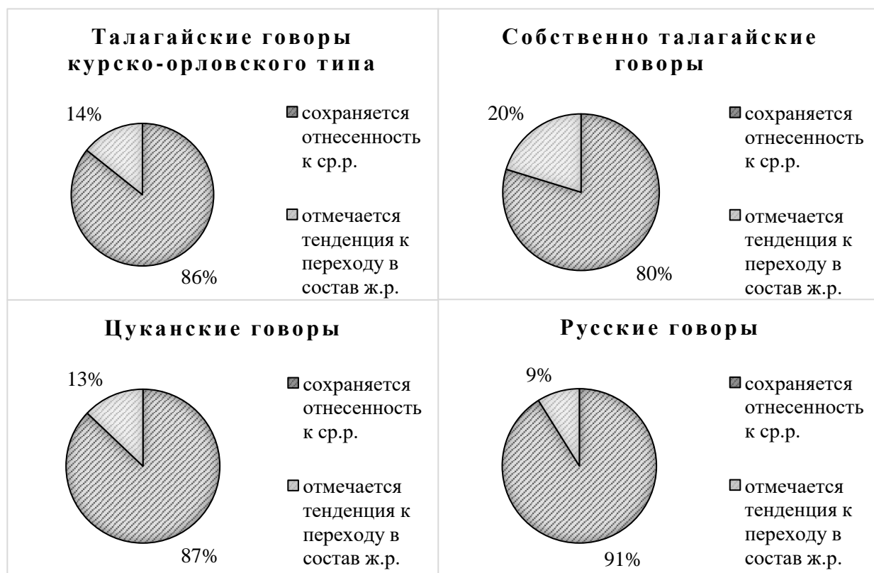
Диаграмма 10. Продуктивность тенденции к разрушению категории среднего рода за счет пополнения состава существительных женского рода в воронежских говорах
