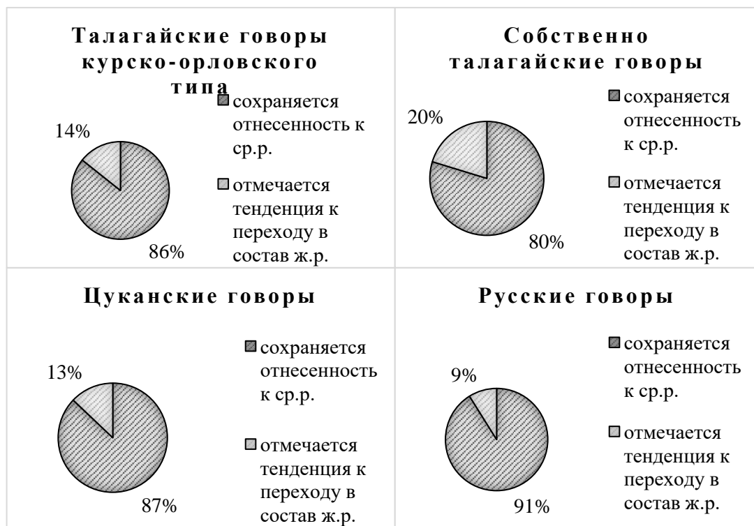
Диаграмма 40. Продуктивность тенденции к разрушению категории среднего рода за счет пополнения состава существительных женского рода в воронежских говорах
