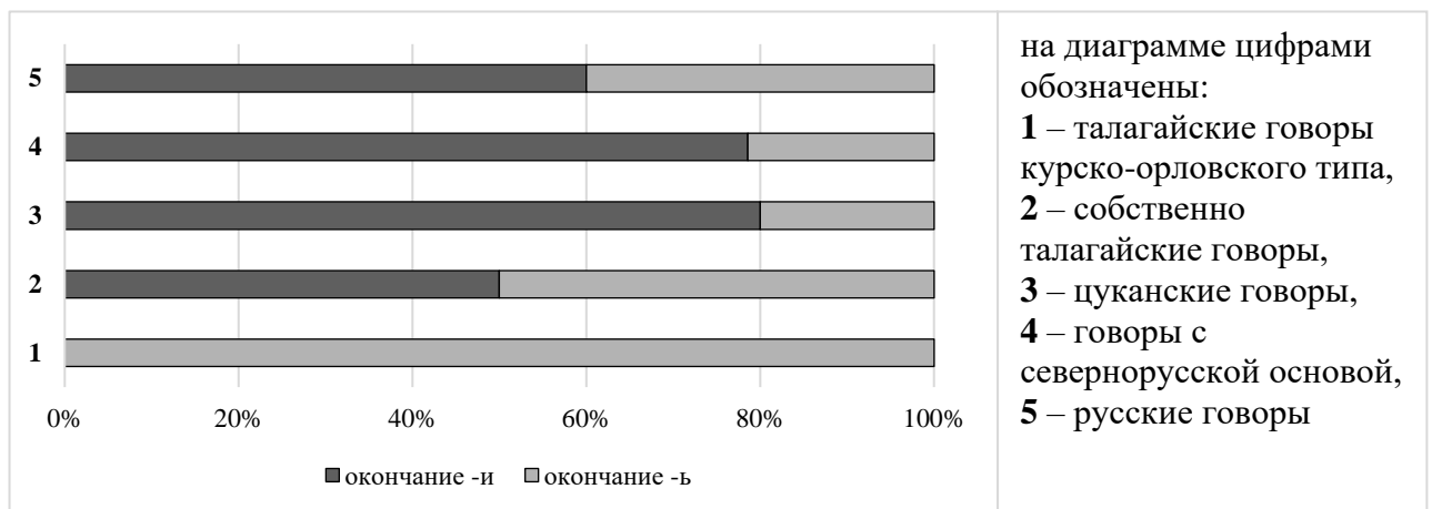
Диаграмма 18. Соотношение вариантов безударного окончания предл.п. ед. ч. 1 скл. существительных в говорах Воронежской области
