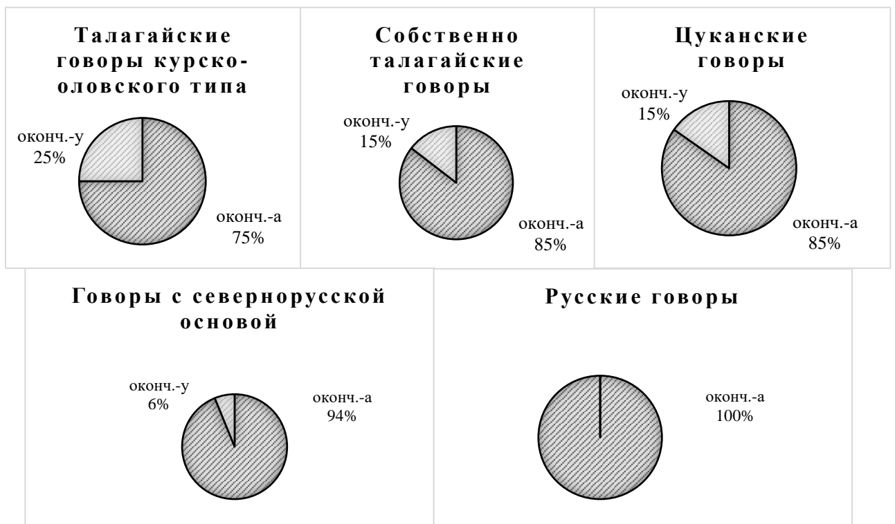
Диаграмма 23. Количественное соотношение вариантных окончаний в род.п. существительных 2 скл. в говорах Воронежской области
