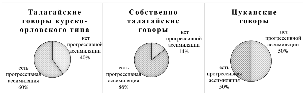
Диаграмма 16. Изменения заднеязычного согласного в результате прогрессивной ассимиляции по мягкости, отраженные в формах вин. п. сущ. 1 скл. в говорах Воронежской области
