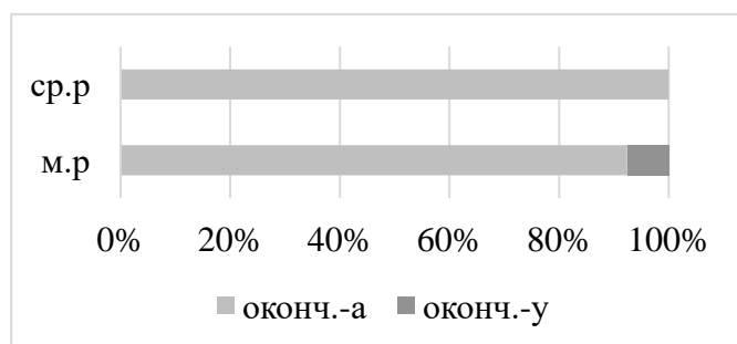
Диаграмма 27. Соотношение вариантных окончаний род. п. сущ. 2 склонения в говорах с севернорусской основой
