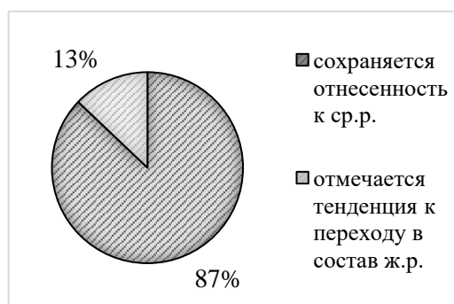
Диаграмма 6. Существительные ср.р. в цуканских говорах
