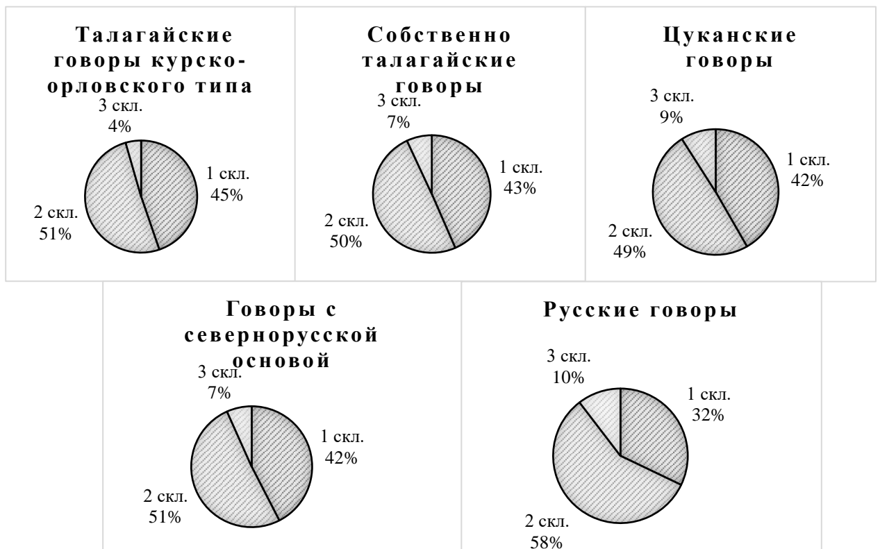
Диаграмма 13. Распределение существительных по типам склонения в говорах Воронежской области
