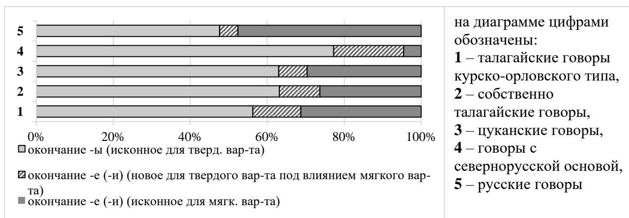
Диаграмма 38. Взаимодействие твердого и мягкого вариантов в род. п. 1-го скл. в говорах Воронежской обл.
