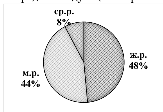
Диаграмма 3. Распределение существительных в ед.ч. по родам в говорах Воронежской области
