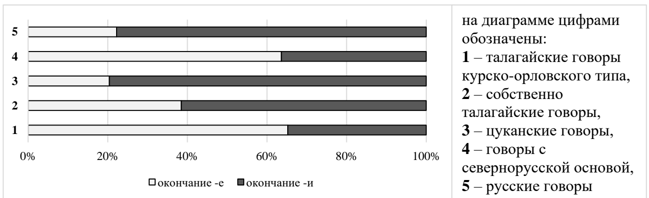
Диаграмма 29. Соотношение вариантов безударных окончаний пр.п. сущ. 2 склонения в говорах Воронежской области
