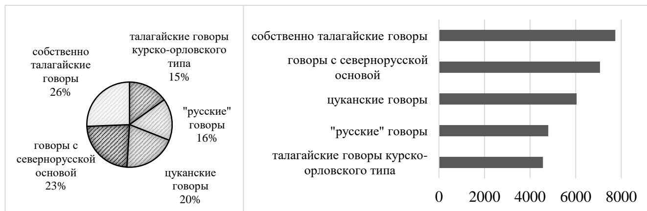
Диаграмма 1. Соотношение подкорпусов диалектных текстов разных типов говоров Воронежской области в составе анализируемого корпуса
