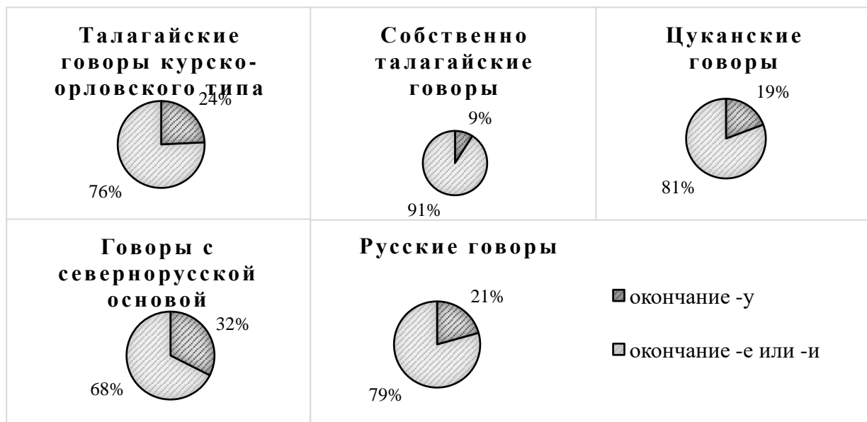
Диаграмма 28. Соотношение вариантных окончаний сущ. 2 склонения в предложном падеже в говорах Воронежской области
