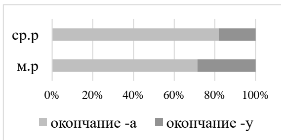
Диаграмма 24. Соотношение вариантных окончаний род. п. сущ. 2 скл. в талагайских говорах курско-орловского типа
