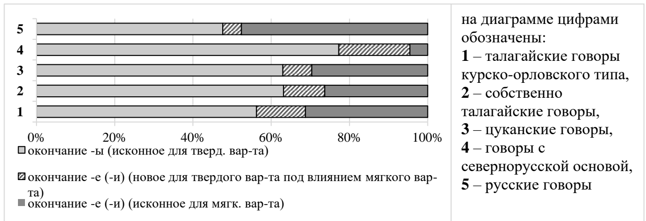
Диаграмма 21. Взаимодействие твердого и мягкого вариантов в род. п. 1-го скл. в говорах Воронежской обл.
