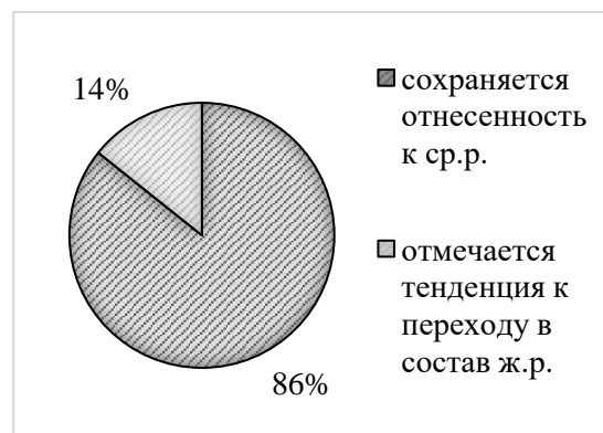
Диаграмма 4. Существительные ср.р. в талагайских говорах курско-орловского типа
