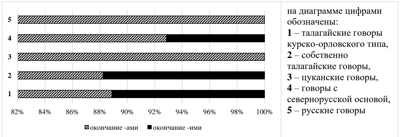
Диаграмма 36. Окончания твор.п. мн.ч. существительных в говорах Воронежской области
